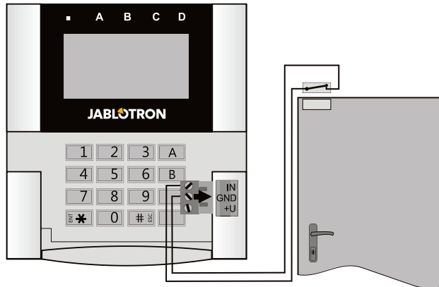
Rysunek 2: Podłączenie styku magnetycznego
