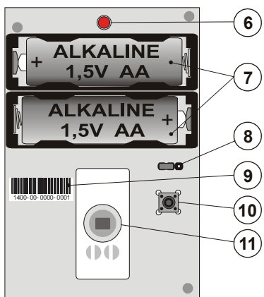
Rysunek: 6 – czerwony wskaźnik aktywacji czujki; 7 – bateria; 8 – zworka zabezpieczeniowa; 9 – kod produkcji; 10 – styk anti-sabotażowy; 11 – sensor PIR;
