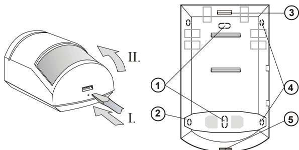
Rysunek: 1 – otwory do montażu ściennego; 2, 4 – otwory do montażu w narożniku; 3 – zatrzask PCB; 5 – zatrzask pokrywy
