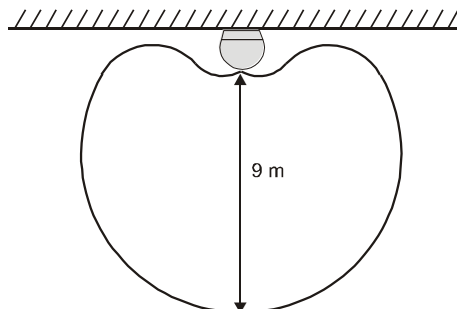
Charakterystyka działania czujnika zbitcia szyby
