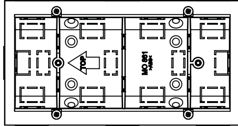
M Montážní otvor Mounting hole X=70/Y=136
