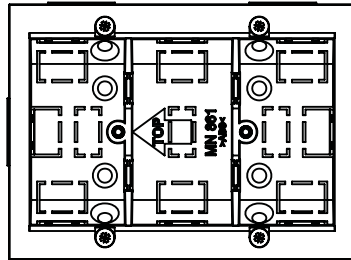
S Montážní otvor Mounting hole X=70/Y=96
